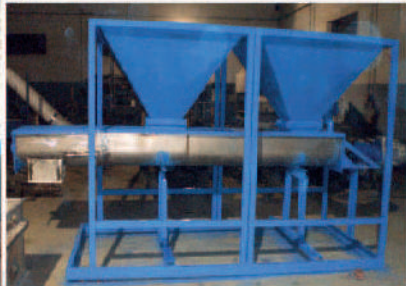
Vis Inox pour grinion
